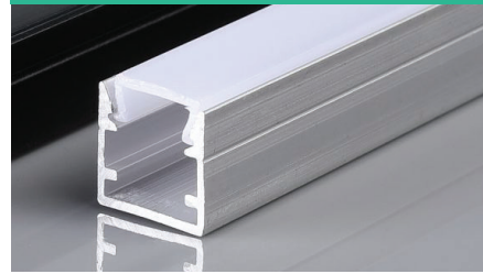
XT-326 Size : 2m*5*13MM
